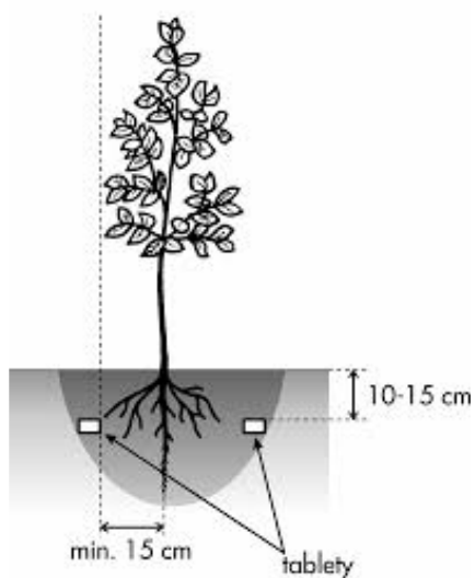
obr. 1 – spôsob umiestňovania tabletového hnojiva do úrovne koreňov vysádzaných drevín (nie pod korene) alebo na okraj výsadbovej jamky (nie však bližšie ako 15 cm ku kmeňku a maximálne 10 cm od priemeru koruny)
