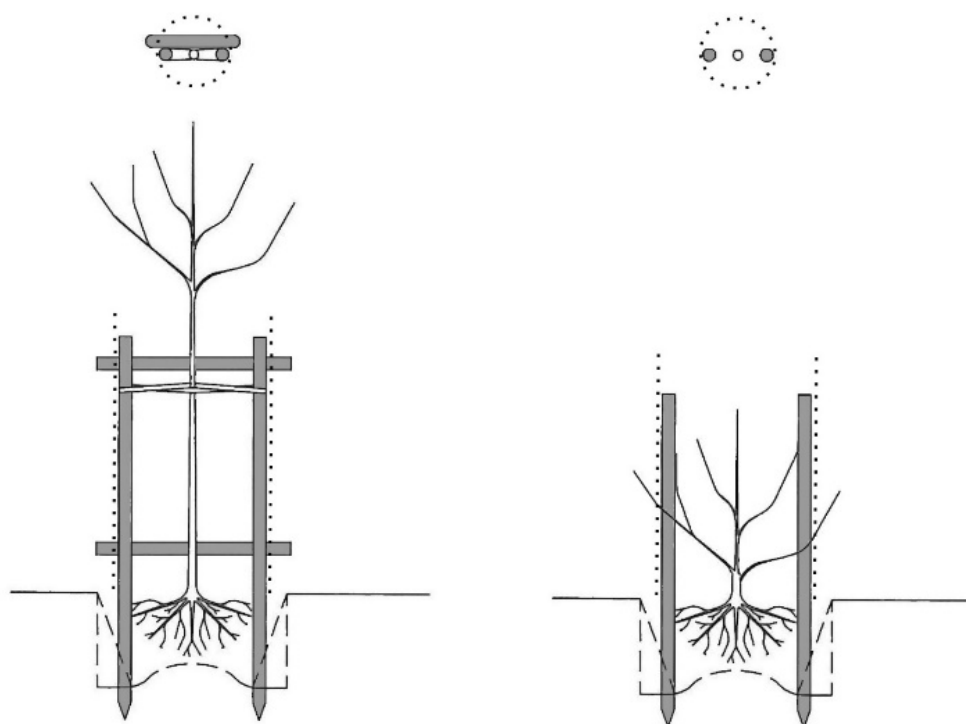
obr. 2 – spôsob umiestnenia nadzemného kotvenia drevín a mechanickej ochrany drevín proti ohryzu - koly sa osadia do vykopanej jamky a umiestnia sa v hĺbke 40-50 cm do kompaktného (prírodného) terénu; pri vzrastlých sadeniciach (vľavo) sa koly vzájomne priečne stabilizujú priečkami v hornej a dolnej časti; pletivo sa upevní ku vonkajšej strane kolov
