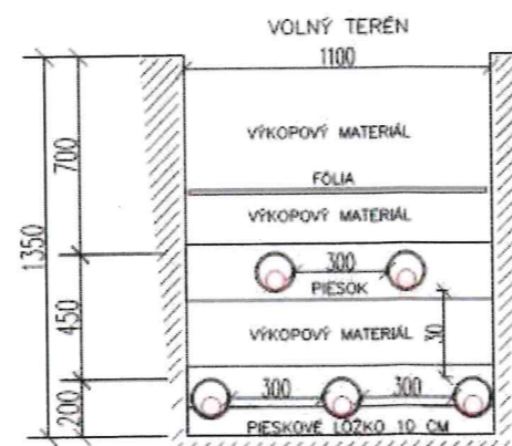
REZ ULOŽENIA NN PRÍPOJKY
